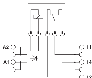
Diagrama eléctrico
